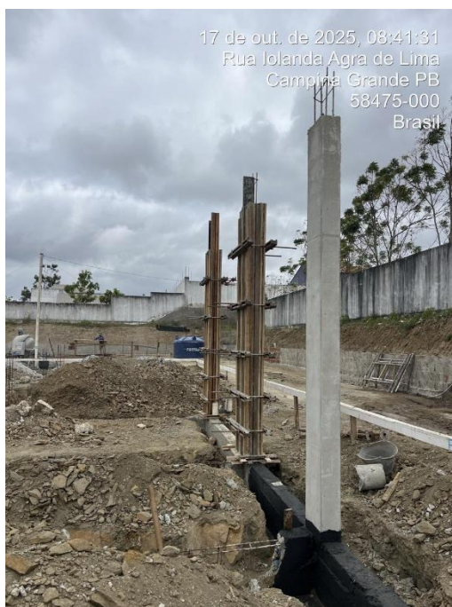
MONTAGEM E DESMONTAGEM DE FORMAS DE PILARES
