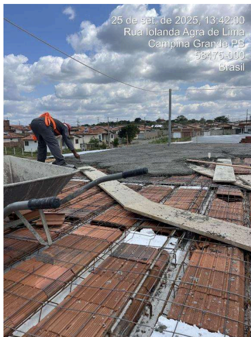
CONCRETAGEM DE LAJE PRE-MOLDADA
