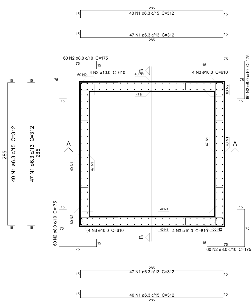
CORTE HORIZONTAL
