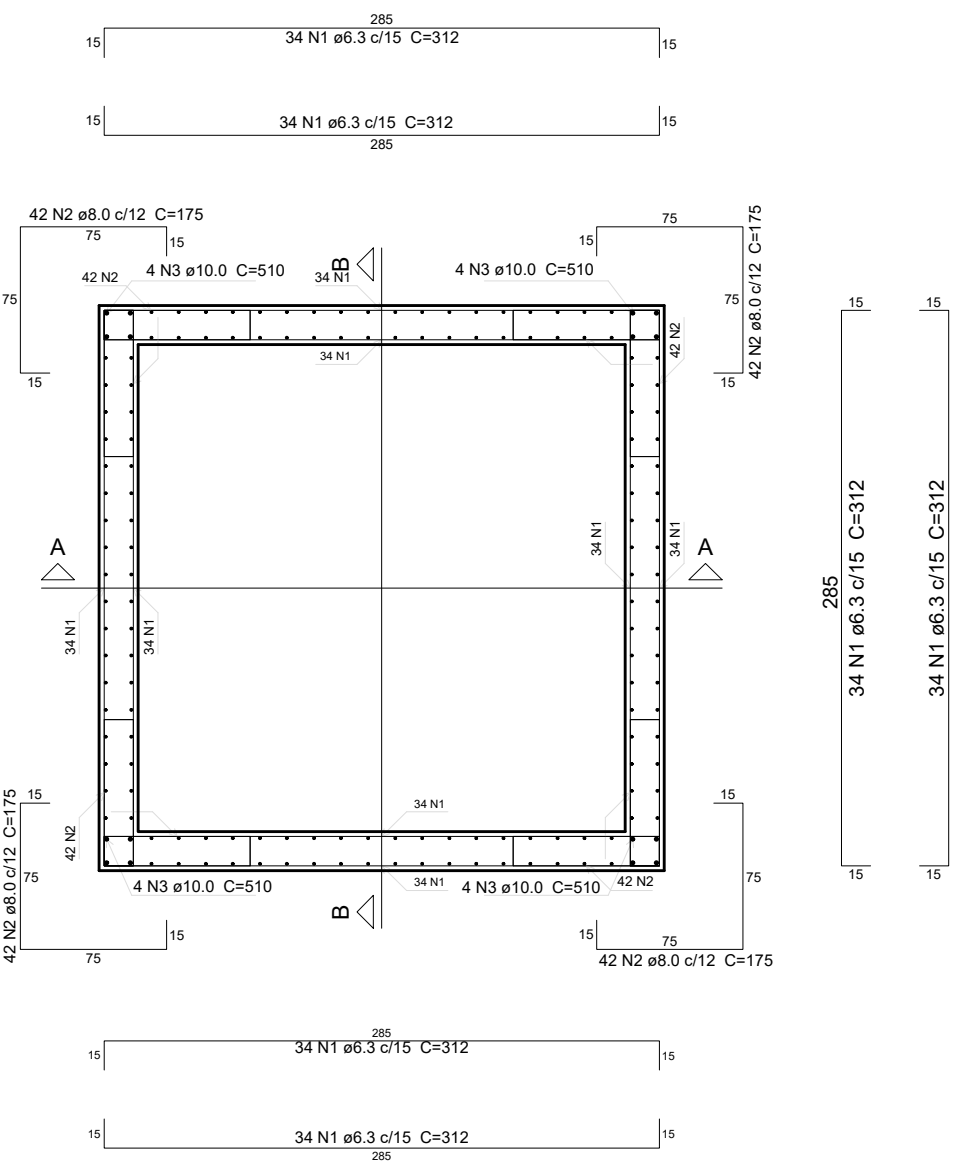
CORTE HORIZONTAL
