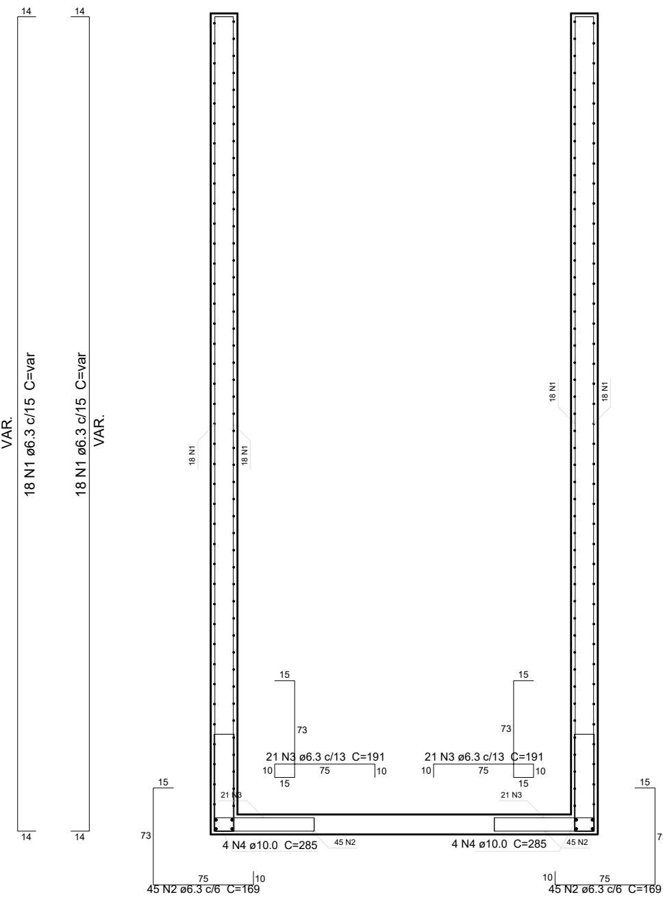
CORTE A-A
