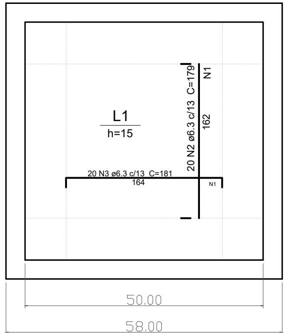
ARMAÇÃO NEGATIVA LAJE DE FUNDO (0.0)
