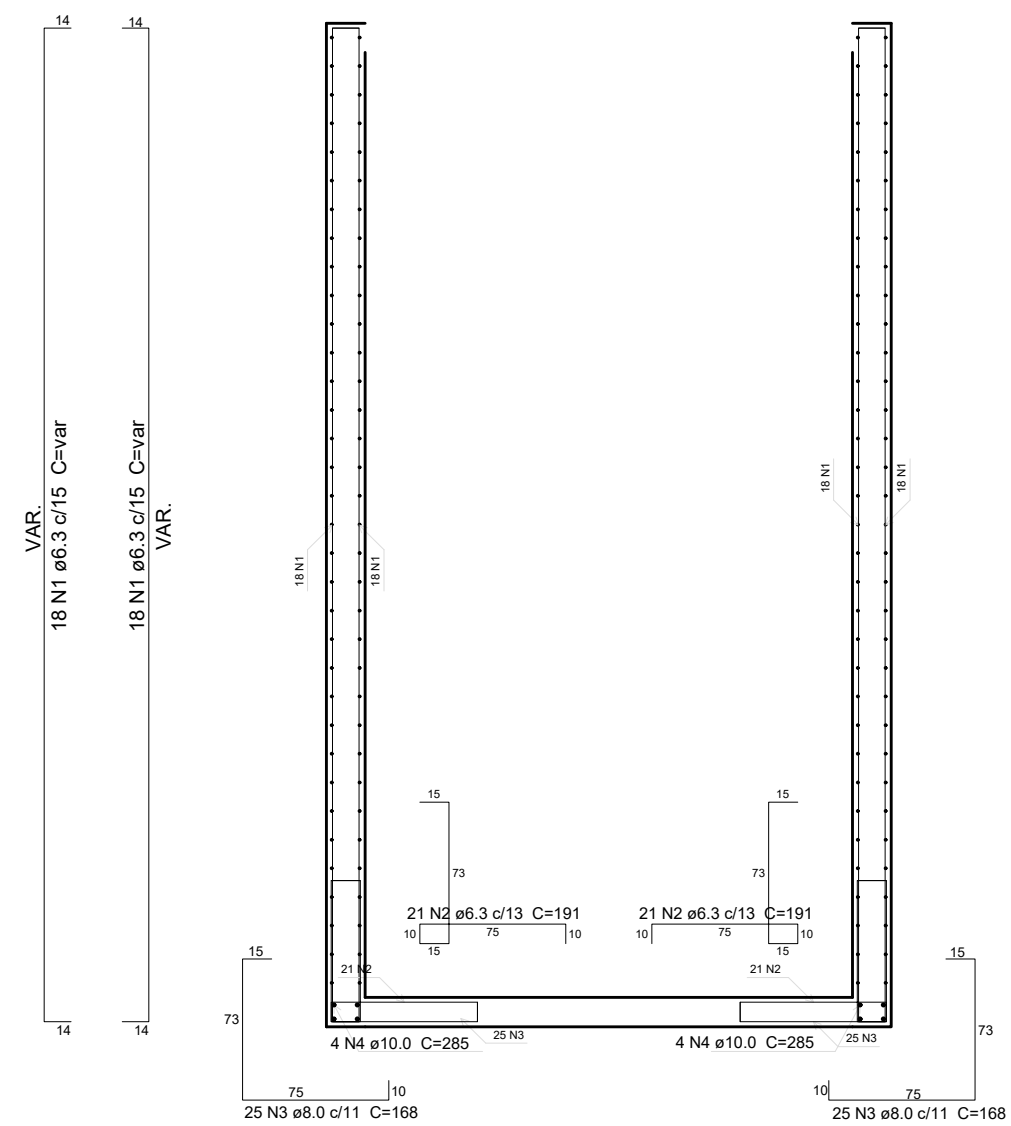
CORTE B-B
