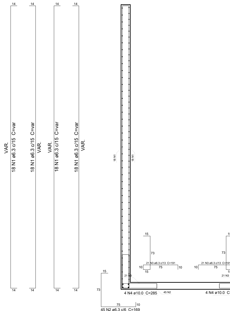
CORTE B-B
