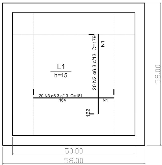
ARMAÇÃO NEGATIVA LAJE DE FUNDO (0.0)
