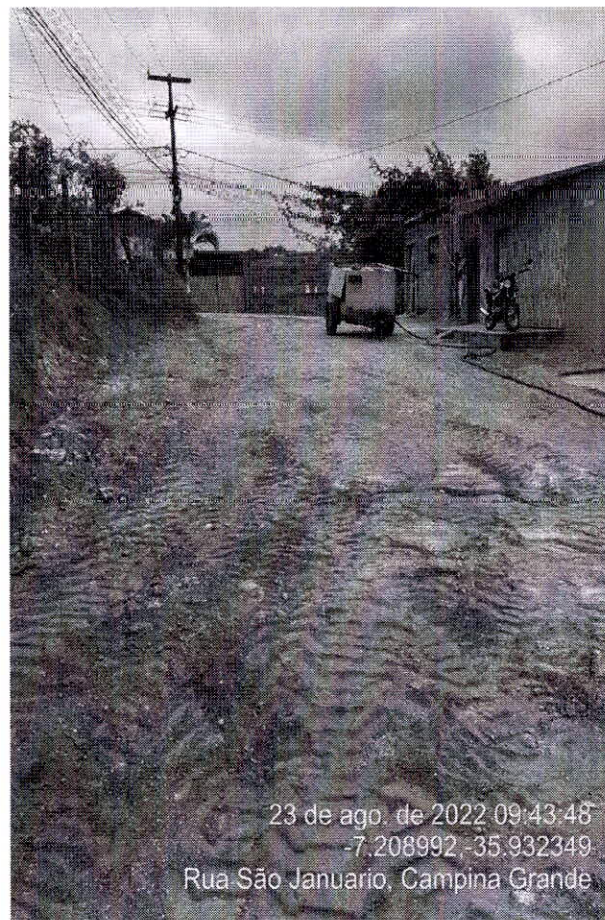
Fotos 04, 05 e 06 – Escavação de material de Terceira categoria
