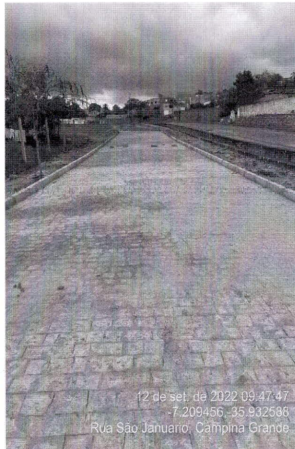
Fotos 13, 14 e 15 – Pavimentação em paralelepípedos
