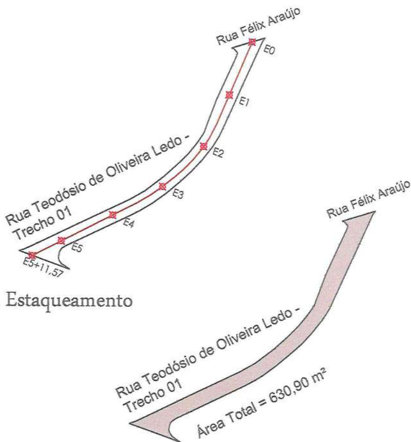
02 - Planta Baixa com Pavimentação Asfáltica (Capa)
