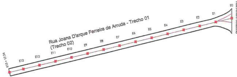
01 - Planta Baixa Estaqueamento
