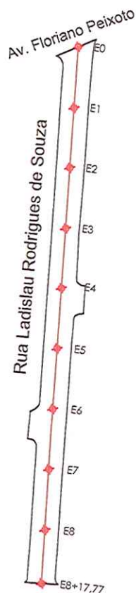
01 - Planta Baixa Estaqueamento
