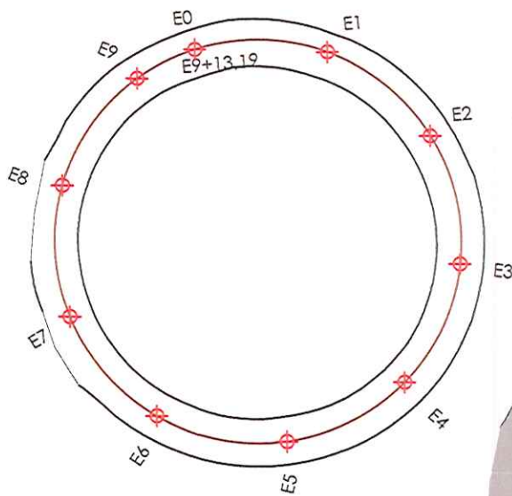
01 - Planta Baixa Estaqueamento
