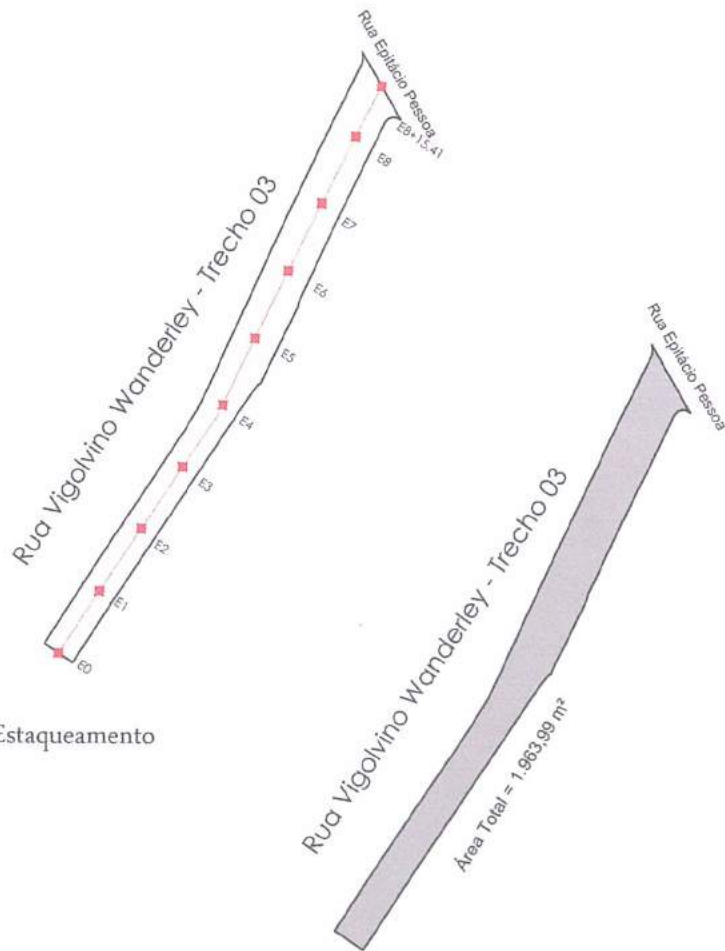
02 - Planta Baixa com Pavimentação Asfáltica (Capa)
