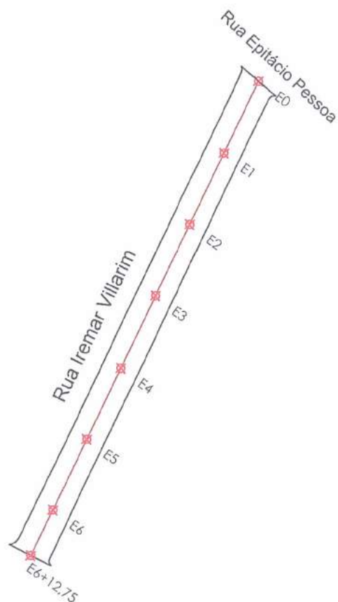
01 - Planta Baixa Estaqueamento
