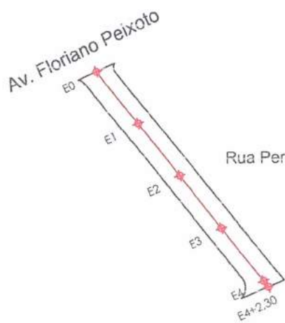
01 - Planta Baixa Estaqueamento
