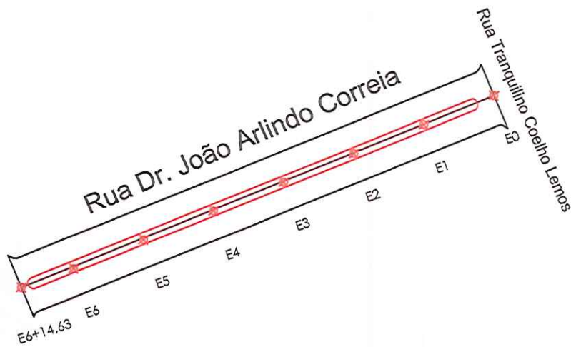
01 - Planta Baixa Estaqueamento
