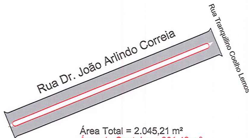
01 - Planta Baixa Estaqueamento
